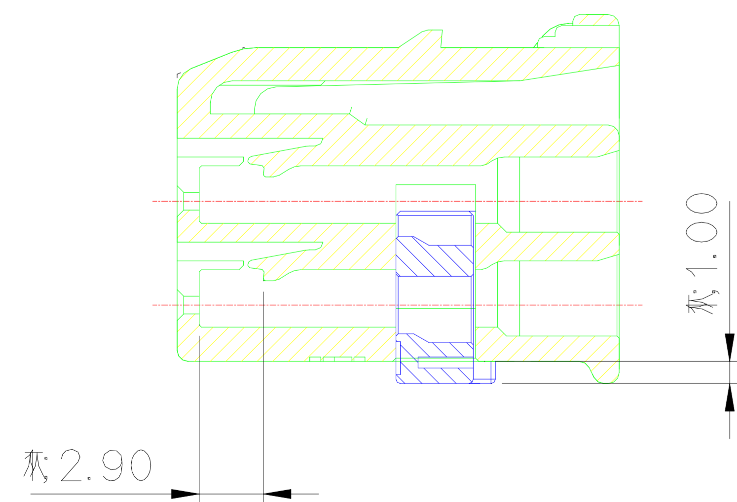
SECTION A-A
