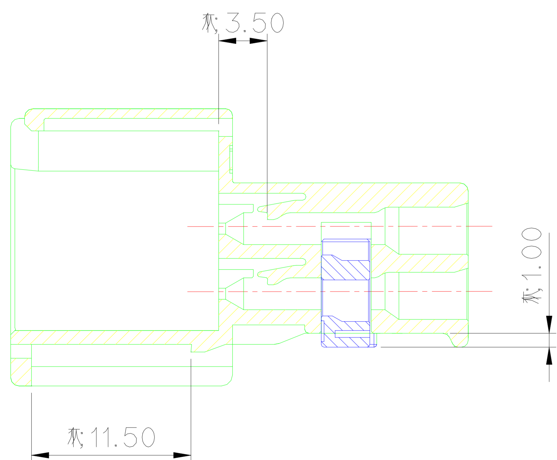
SECTION A-A
